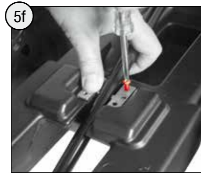
4x D Ø4 x 16
